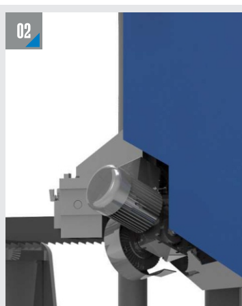
ПРИВОДНАЯ ЩЕТКА ДЛЯ ОЧИСТКИ ПОЛОТНА
